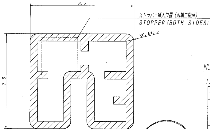
断面拡大図 SECT. DETAIL
