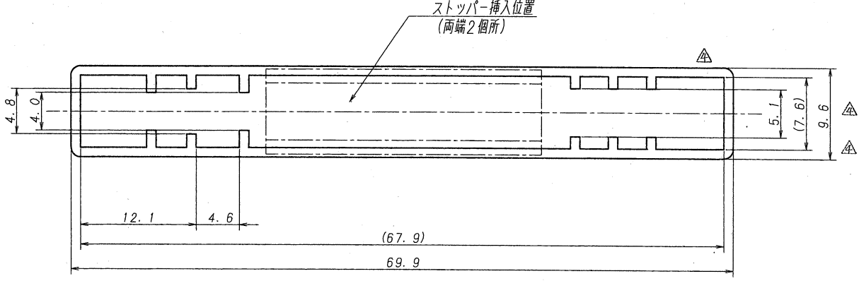
断面拡大図
