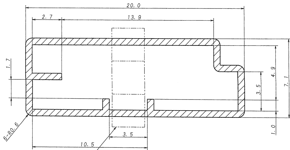
断面拡大図
