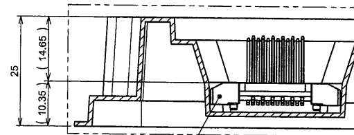
SECT A-A
