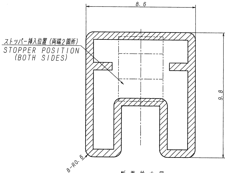
断面拡大図 SECT. DETAILS
