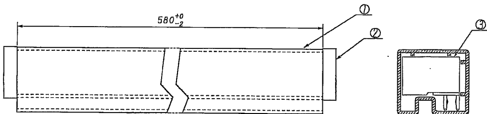
断面拡大図 SECT. DETAIL
