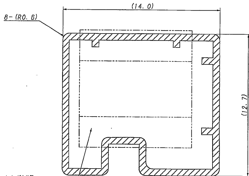
断面拡大図 SECT. DETAIL
