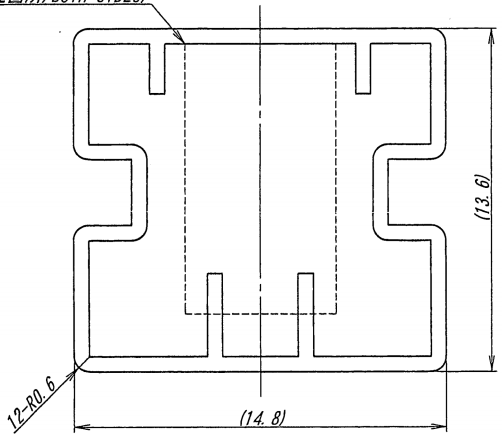
断面拡大図 SECT. DETAIL
