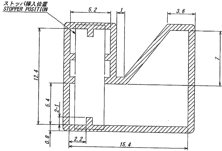
断面拡大図 DETAIL SECTION
