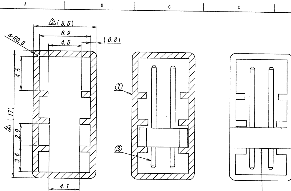
断面拡大図 SECT. DETAIL
