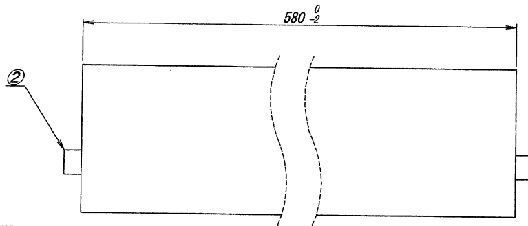
ストッパー位置 (両端2ヶ所) STOPPER POSITION (BOTH SIDE)
