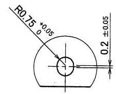
詳細 H スケール 4:1
