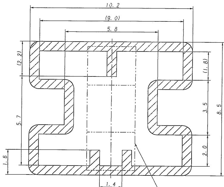
断面拡大図 SECT. DETAIL
