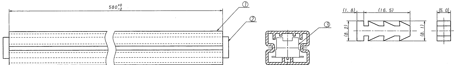
断面拡大図 CROSS SECTION
