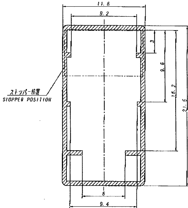
断面図 SECT. DETAIL
