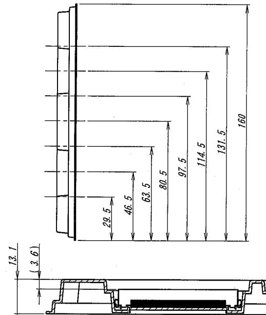
SECT D-D
