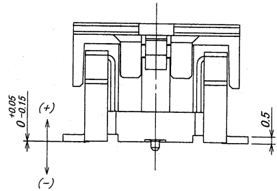
キャップ無し/WITH OUT CAP
