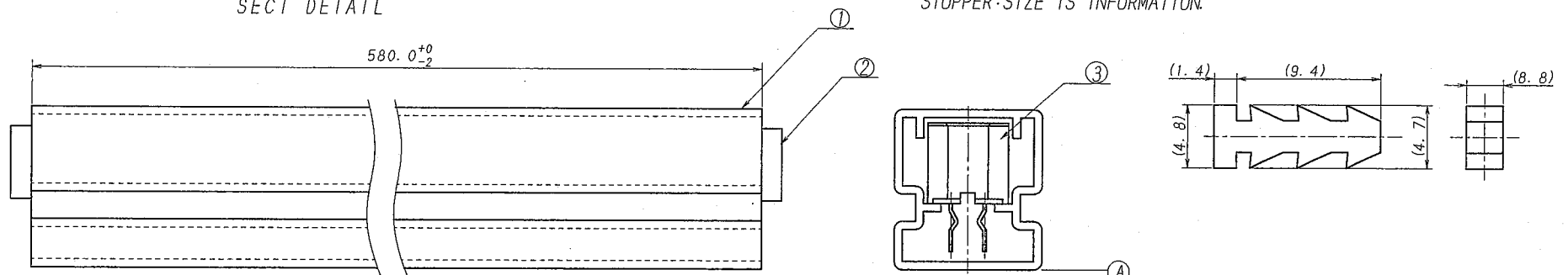
断面拡大図 SECT DETAIL
