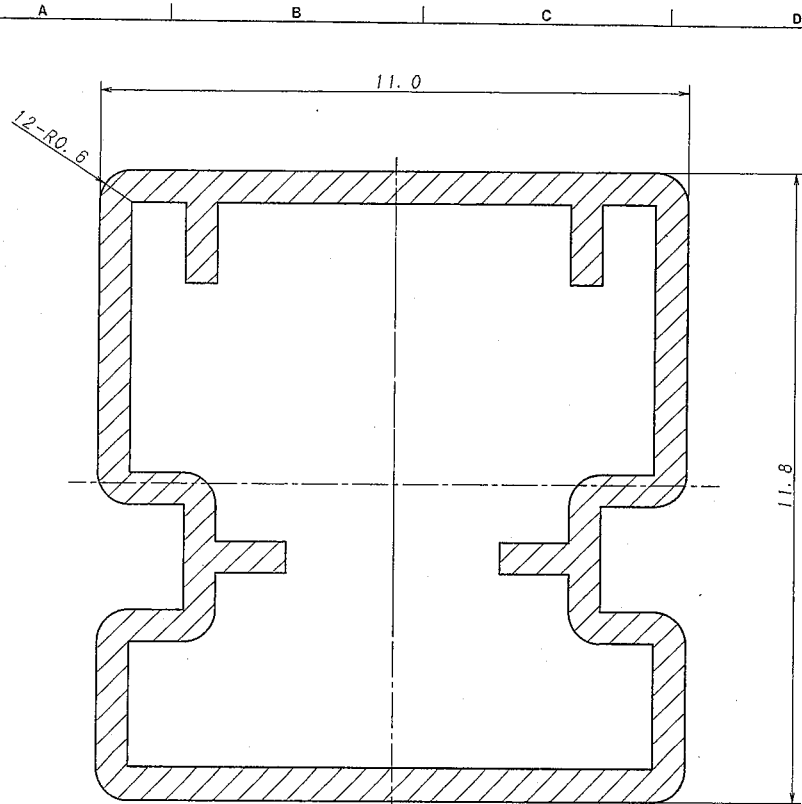
断面拡大図 SECT DETAIL
