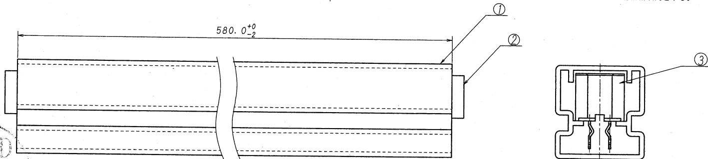
断面拡大図 SECT DETAIL
