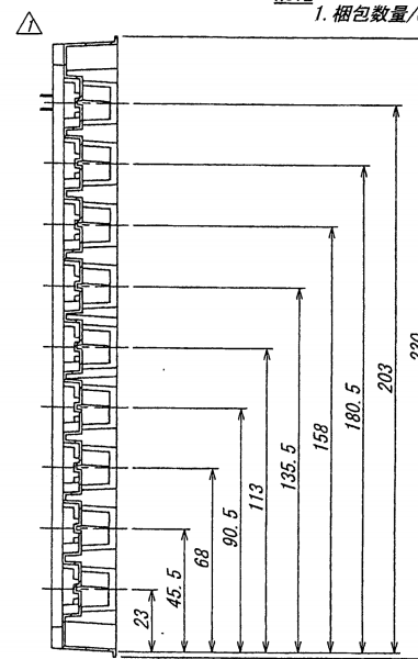
SECT A-A
