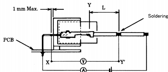
Y-Y 間の抵抗(電線'L'分)を差し引くこと。 Deduct resistance Y-Y(wire'L')from X-Y
